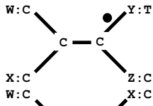
Tree 1: ((WX)(YZ))
