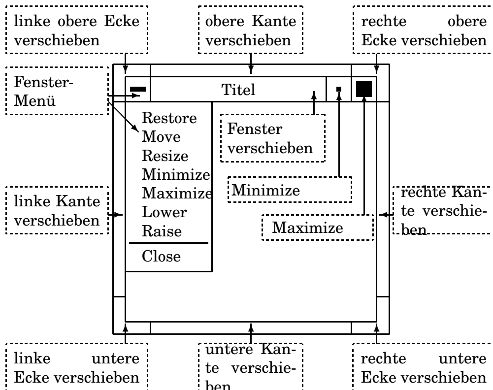
Abb. 2.9: OSF/Motif-Fenster
