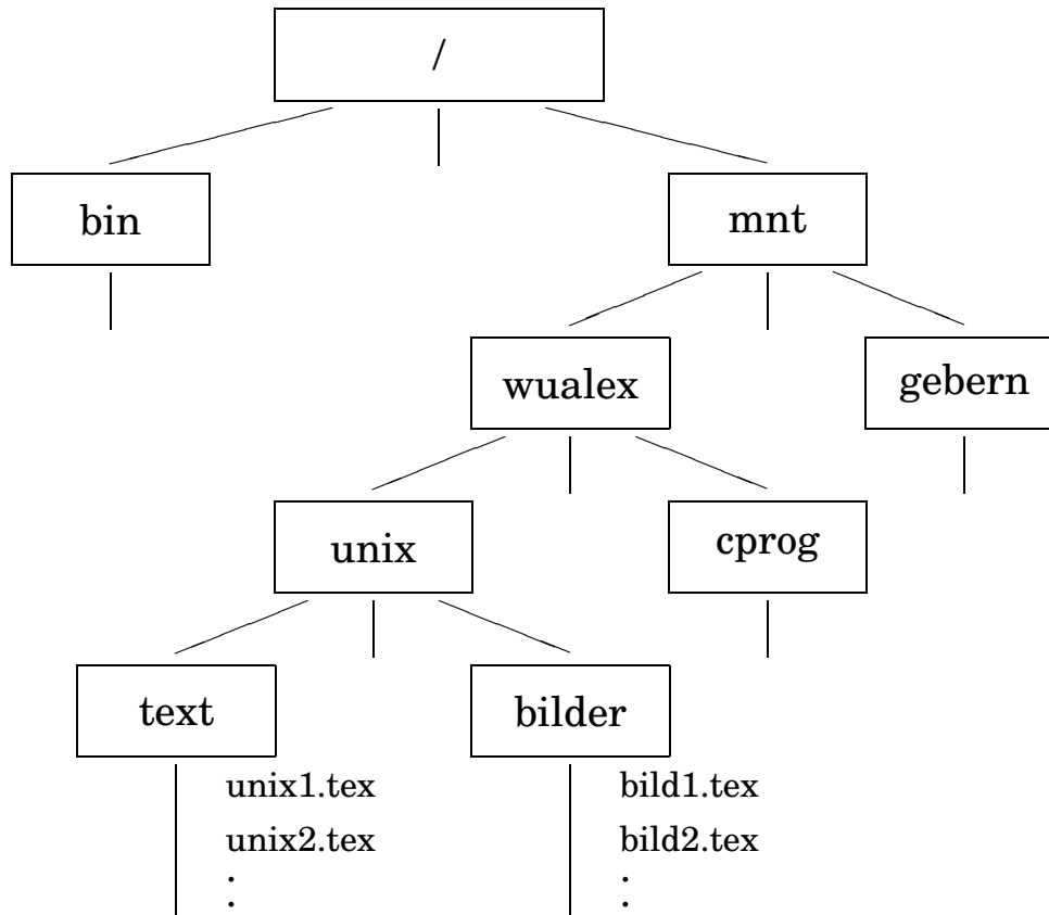
Abb. 2.4: UNIX-Dateihierarchie
